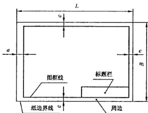
图 4 有装订边图纸(X 型)的图框格式
